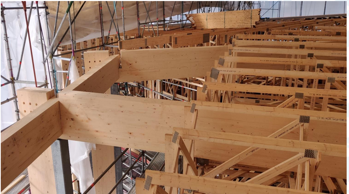
Yläpohjan puurakenteita
